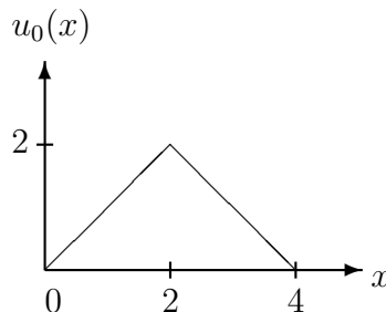
Bild 18 Anfangsfunktion u_0
