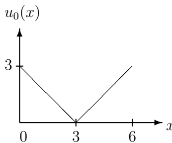
Bild 19 Anfangsfunktion u_0
